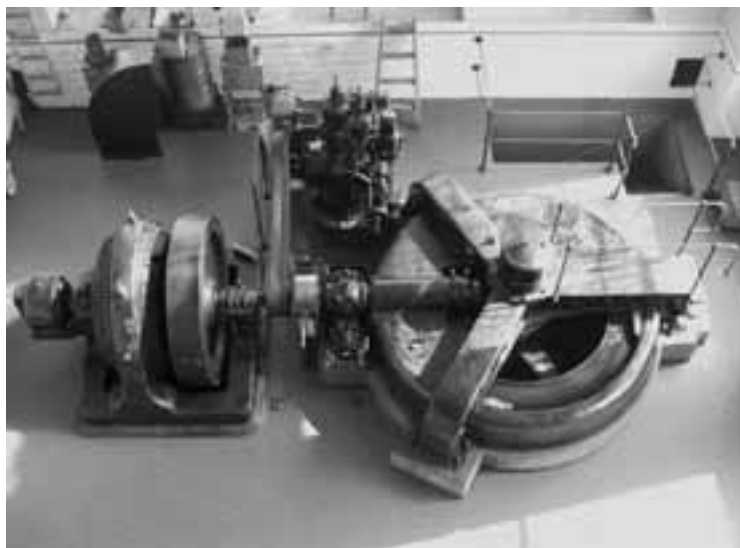
Pohled do stávající strojovny elektrárny
